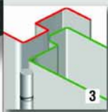
Antidégondage par tenon-mortaise
