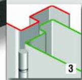
Antidégondage par tenon-mortaise
