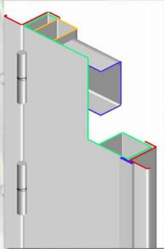
modèle présenté en droite poussante avec anti-panique Push bar JPM 1 point
